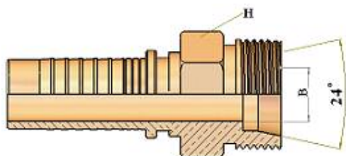
HT11510 METRIC MALE 24° CONE SEAT L.T. DIN 3861
