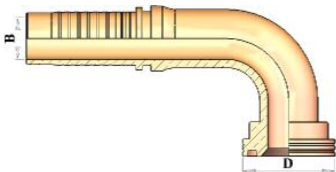
HT23390 90° FLANGE 3000 P.S.I. كوع ٩٠° فلانج قطعة واحدة 3000 P.S.I.
