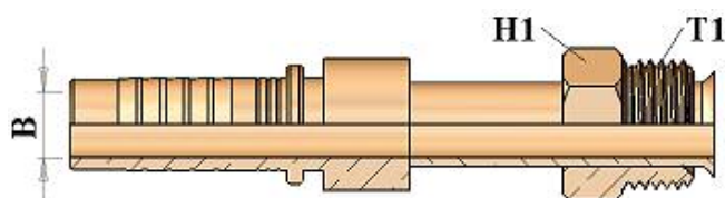
JIC MF-ST مستقيم MF سن أمريكي
