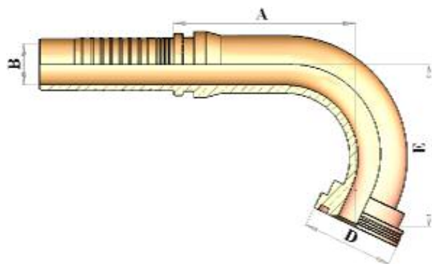
HT233110 110° FLANGE 3000 P.S.I. فلانج قطعة واحدة ١١٠° 3000 P.S.I.
