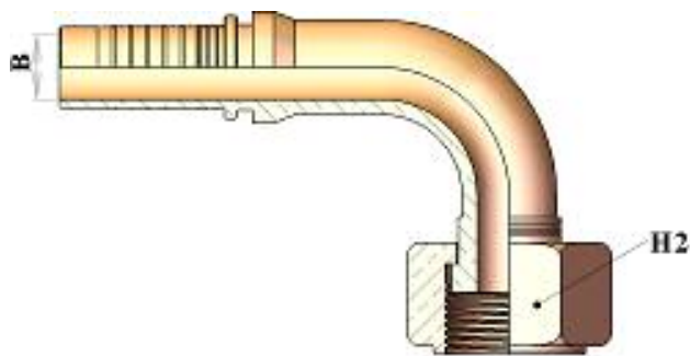
HT22493 90° OFRS FEMALE ORFS ٩٠ كوع
