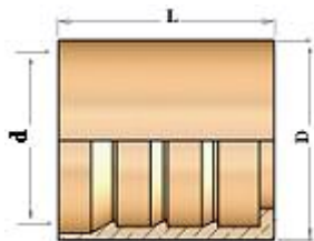
HT00200 SWAGED FERRULE FOR SAE 100 R2A +2ST HOSE SKIVE + 4SP HOSE جلبة (سوكيت) طاقين قشط + ٤ طوق قصير
