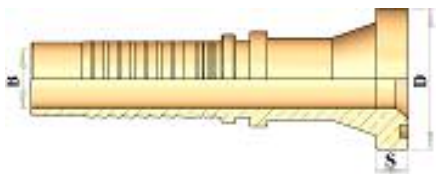
HT23711 L.L LITTLE LONG DROP STRAIGHT FLANGE 6000 P.S.I. 6000 P.S.I. مستقيم فلانج طويل قليلاً قطعة واحدة
