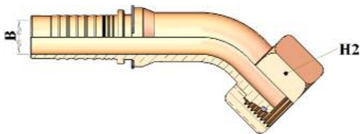
HT21643 45° O’RING METRIC SWEEP ELBOW 24° CONE H.T. DIN 3865
