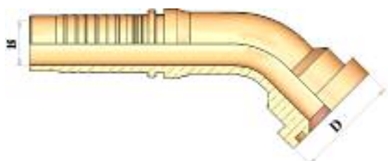
HT23645 45° FLANGE 6000 P.S.I. 6000 P.S.I. نصف كوع ٤٥ درجة قطعة واحدة
