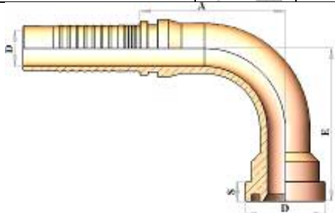
HT23790L.L 90° LITTLE LONG DROP FLANGE 6000 P.S.I. 6000 P.S.I. كوع فلانج ٩٠° طويل قليلاً قطعة واحدة
