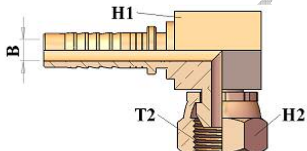
HT20881 90° BSP COMPACT ELBOW كوع BSP طرق
