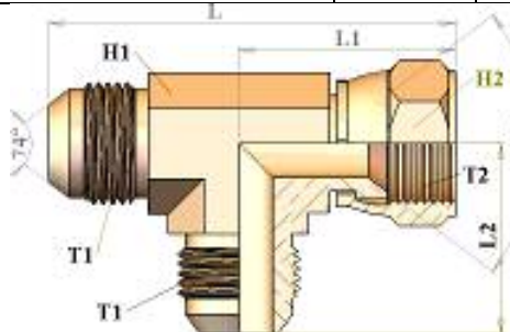
HT722525 RUN TEE ADAPTOR JIC MALE / JIC FEMALE 74° CONE مثلث سن JIC طرف ووسط ذكر وطرف متحرك
