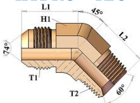
HT532507 45 ELBOW ADAPTOR JIC MALE / BSPT MALE نبل نصف كوع ذكر سن JIC / ذكر سن BSPT
