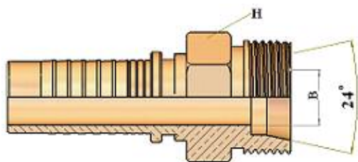
HT11610 O’RING METRIC FEMALE 24° CONE HEAVY DUTY ( H.T) DIN 3865 ذكر متري ٢٤° أعمال ثقيلة
