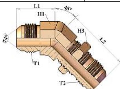
HT532523 45 ELBOW BULKHEAD ADAPTOR JIC MALE 74 CONE نبيل نصف كوع ذكر سن JIC طويل مع عزقة كمنترول / ذكر سن JIC
