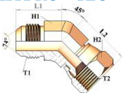
HT552525 45 ELBOW ADAPTOR JIC MALE / JIC FEMALE نبيل نصف كوع متحرك سن JIC / ذكر سن JIC
