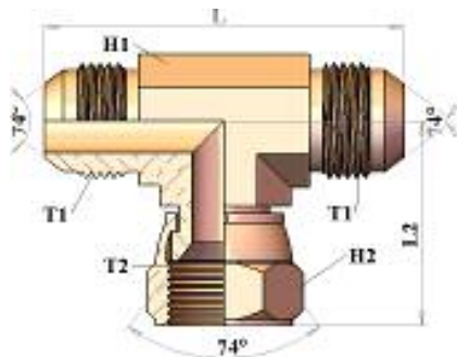
HT712525 UNION TEE ADAPTOR JIC MALE / JIC FEMALE 74° CONE مثلث سن JIC طرفين ذكر وسط متحرك
