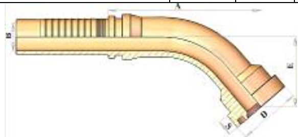
HT23745L.L 45° LITTLE LONG DROP FLANGE 6000 P.S.I. 6000 P.S.I. نصف كوع فلانج ٤٥° طويل قليلاً قطعة واحدة
