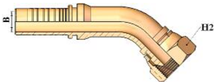
HT22541 45° JIC SWEPT ELBOW 74° CONE نصف كوع ٤٥° سن JIC ٧٤° عزقة كبس
