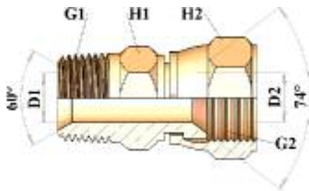
HT520725 STRIGHT ADAPTOR BSPT MALE / JIC FEMALE نبيل متحرك سن JIC / ذكر سن BSPT
