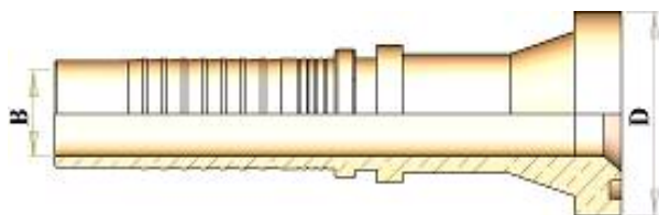
HT23611 STRAIGHT FLANGE 6000 P.S.I. مستقيم فلانج قطعة واحدة 6000 P.S.I.
