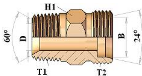
HT500715 STRAIGHT ADAPTOR BSPT MALE / METRIC MALE نبيل ذكر متري / ذكر BSPT
