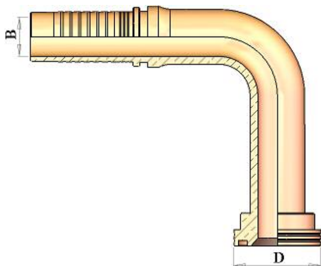
HT23390L 90° LONG DROP FLANGE 3000 P.S.I. كوع فلانج ٩٠° طويل قطعة واحدة 3000 P.S.I.
