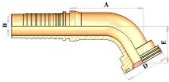
HT23360 60° FLANGE 3000 P.S.I. فلانج زاوية ٦٠° قطعة واحدة 3000 P.S.I.
