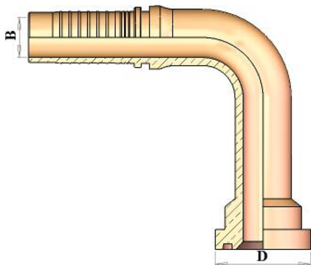
SUPER CAT HT23990L 90° LONG DROP FLANGE 9000 P.S.I. كوع فلانج ٩٠° طويل قطعة واحدة 9000 P.S.I.
