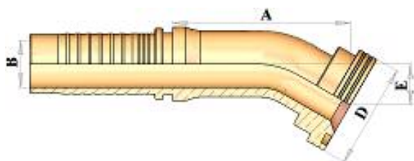
HT23330 30° FLANGE 3000 P.S.I. فلانج زاوية ٣٠ ° قطعة واحدة 3000 P.S.I.
