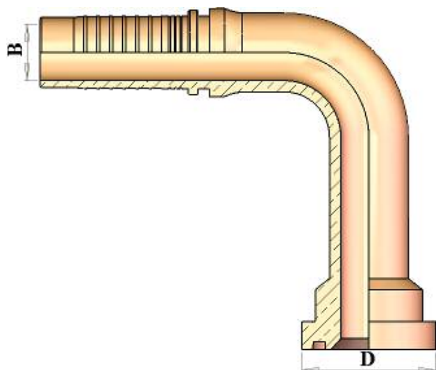
HT23690L 90° LONG DROP FLANGE 6000 P.S.I. كوع فلانج ٩٠° طويل قطعة واحدة 6000 P.S.I.
