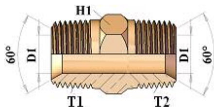
HT500707 STRAIGHT ADAPTOR BEST MALE / BEST MALE نبيل ذكر سن BSPT
