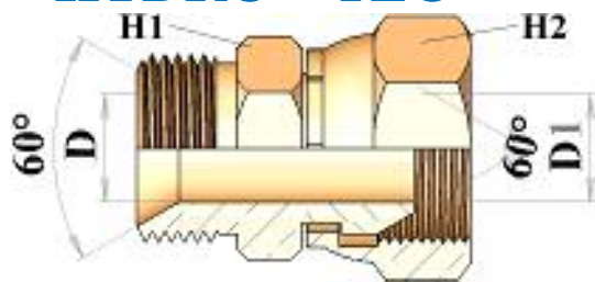
HT520405 STRAIGHT ADAPTOR BSP MALE / BSP FEMALE (C/B NUT) نبل أنثى سن / ذكر مسدس صغير سن BSP
