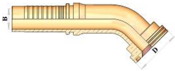
HT23345 45° FLANGE 3000 P.S.I. نصف كوع ٤٥° فلانج قطعة واحدة 3000 P.S.I.
