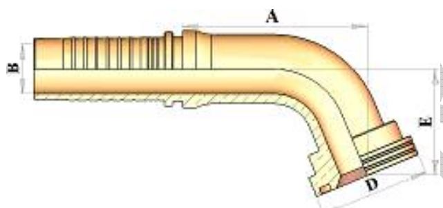
HT23367 67.5° FLANGE 3000 P.S.I. فلانج زاوية ٦٧.٥° قطعة واحدة 3000 P.S.I.
