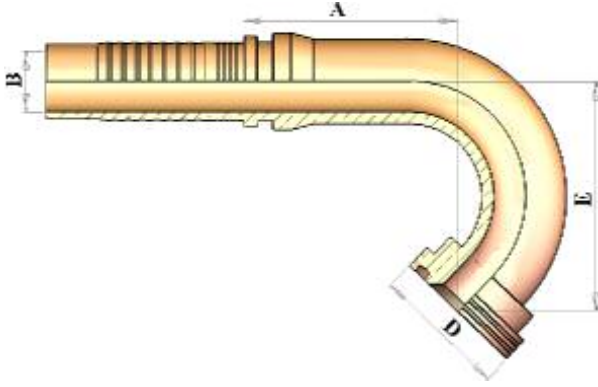
HT233135 135° FLANGE 3000 P.S.I. فلانج قطعة واحدة ١٣٥° 3000 P.S.I.
