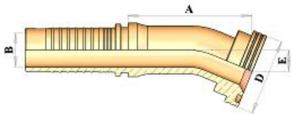
HT23322 22.5° FLANGE 3000 P.S.I. فلانج زاوية ٢٢.٥ ° قطعة واحدة 3000 P.S.I.
