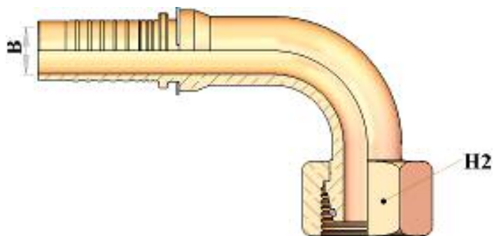
HT21593 90° O’RING METRIC SWEPT ELBOW 24° CONE L.T. DIN 3865 كوع ٩٠ متري ٢٤ بسيلة
