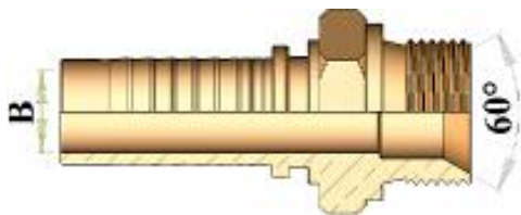
HT10510 BSP MALE PARALLEL 60° CONE SEAT ذكر سن BSP مع مركز سيلة كونيك 60°
