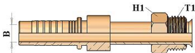
METRIC MF-ST مستقيم MF سن متري
